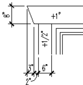
HEADER DTL.
