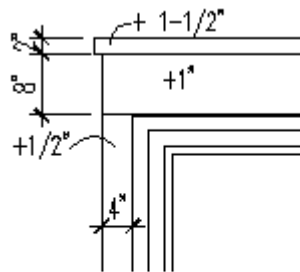
HEADER DTL
